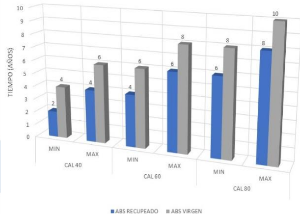
DURABILIDAD (AÑOS) MÓDULOS DE SEDIMENTACION ABS
